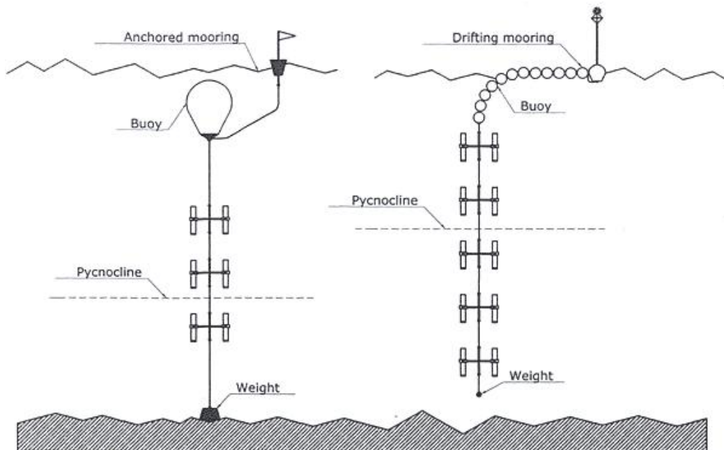
丹麦 KC-Denmark 公司多通道沉积物捕集器工作示意图
